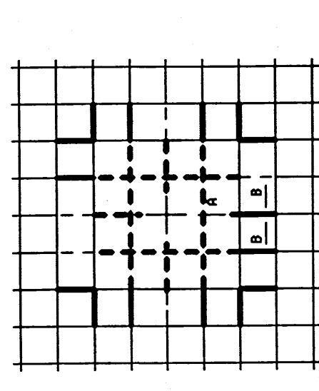
DETALLE DE ARMADO A CORTANTE
